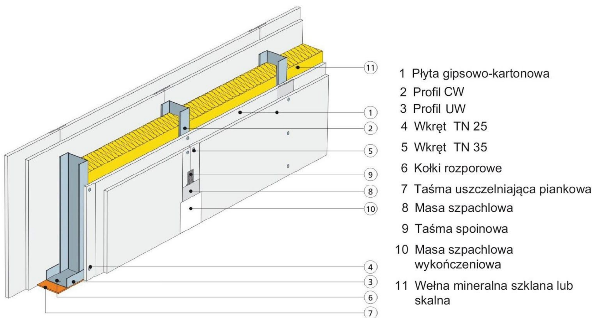
Projektowana ściana działowa gr. 15 cm
